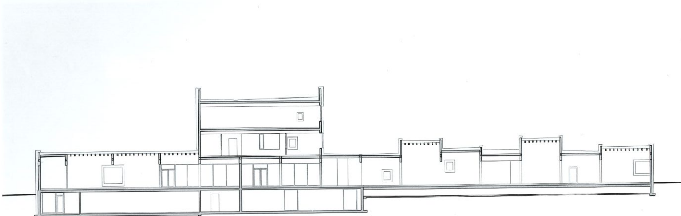
Coupe longitudinale montrant les réserves au sous-sol, les deux étages de bureaux et les espaces d'exposition au rez-de-chaussée
